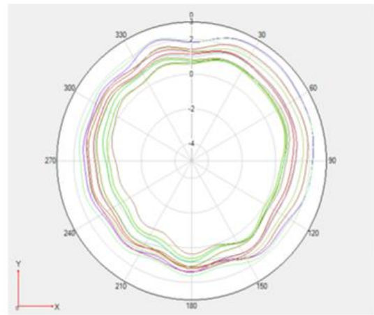
天线的垂直面方向图（V面）
