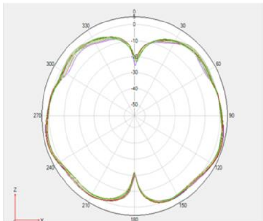
天线的水平面方向图（H面）
